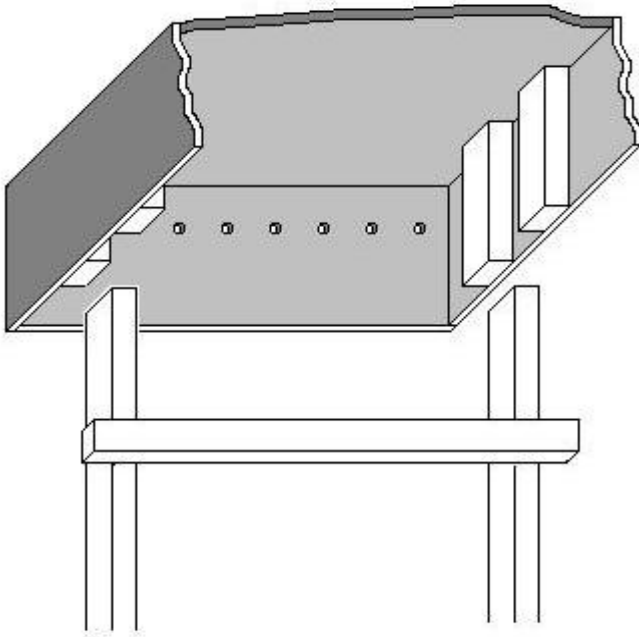
Abbildung SEQ Abbildung 1 ARABIC 1: Verbindung des Modulkastens mit dem Untergestell
