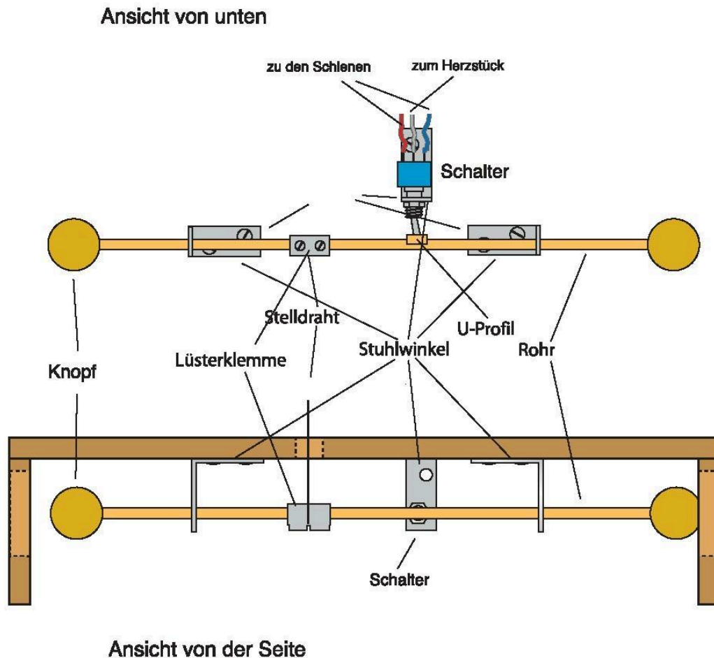
Abbildung 4: Mechanischer Weichenantrieb
